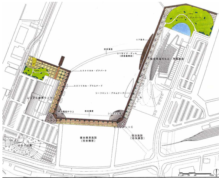
(図5-1) 小名浜港1・2号埠頭地区緑地の基本計画図
